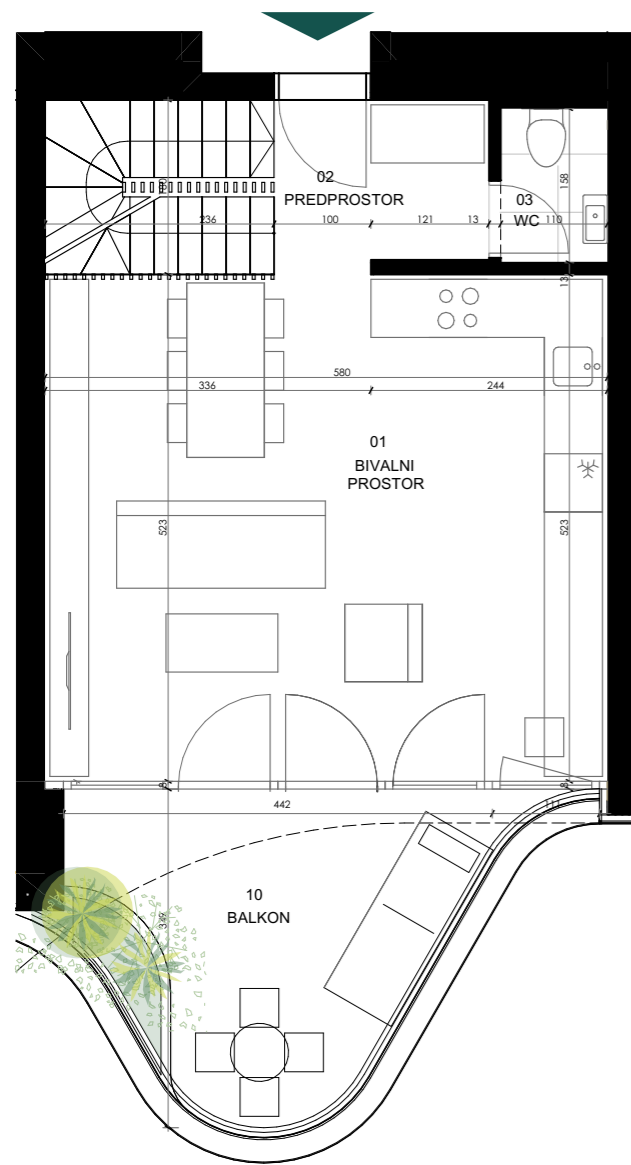
PRVI NIVO STANOVANJA (TRETJA ETAŽA)
