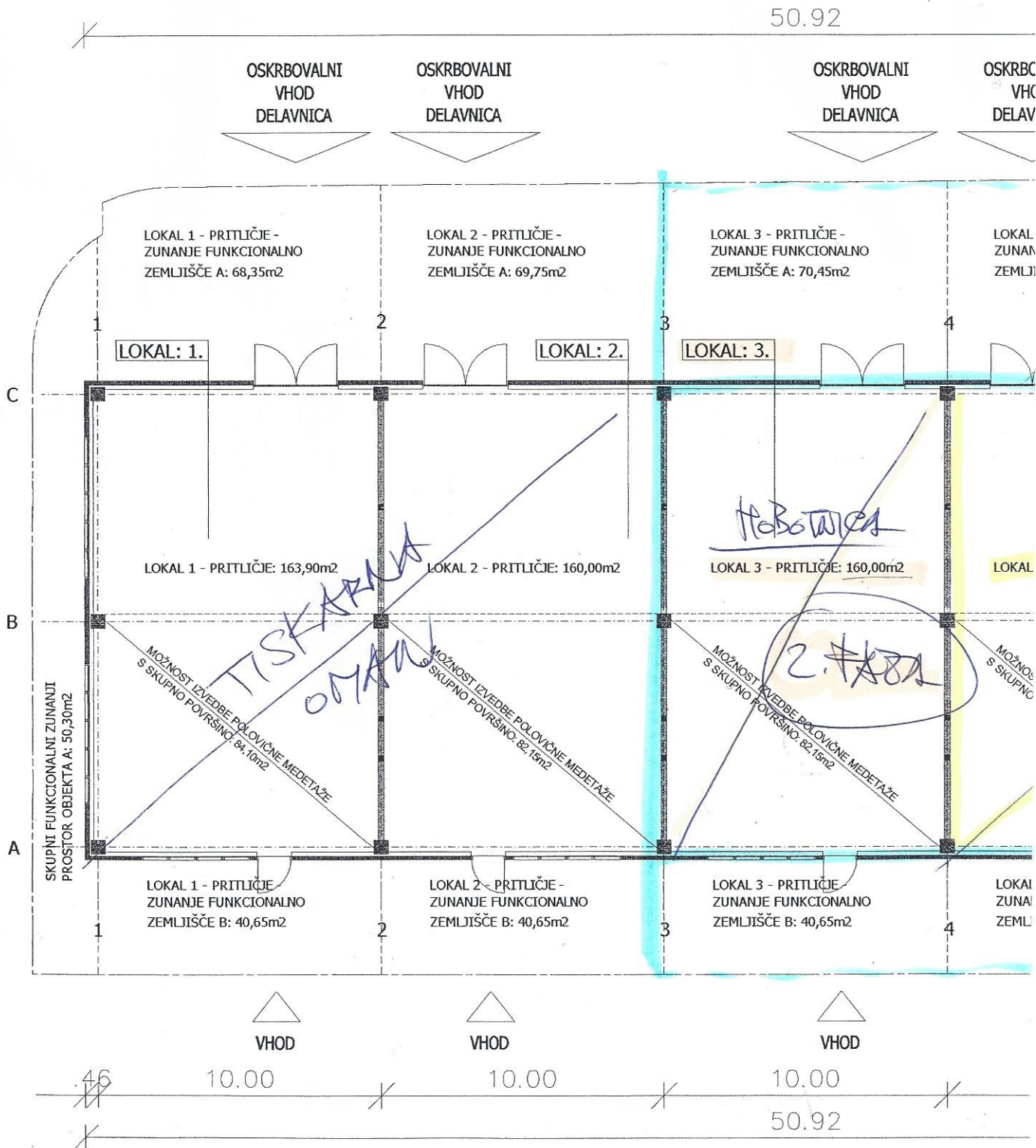
TLORIS PRITLIČJA OBJEKTA 3-3 MERILO 1:200
