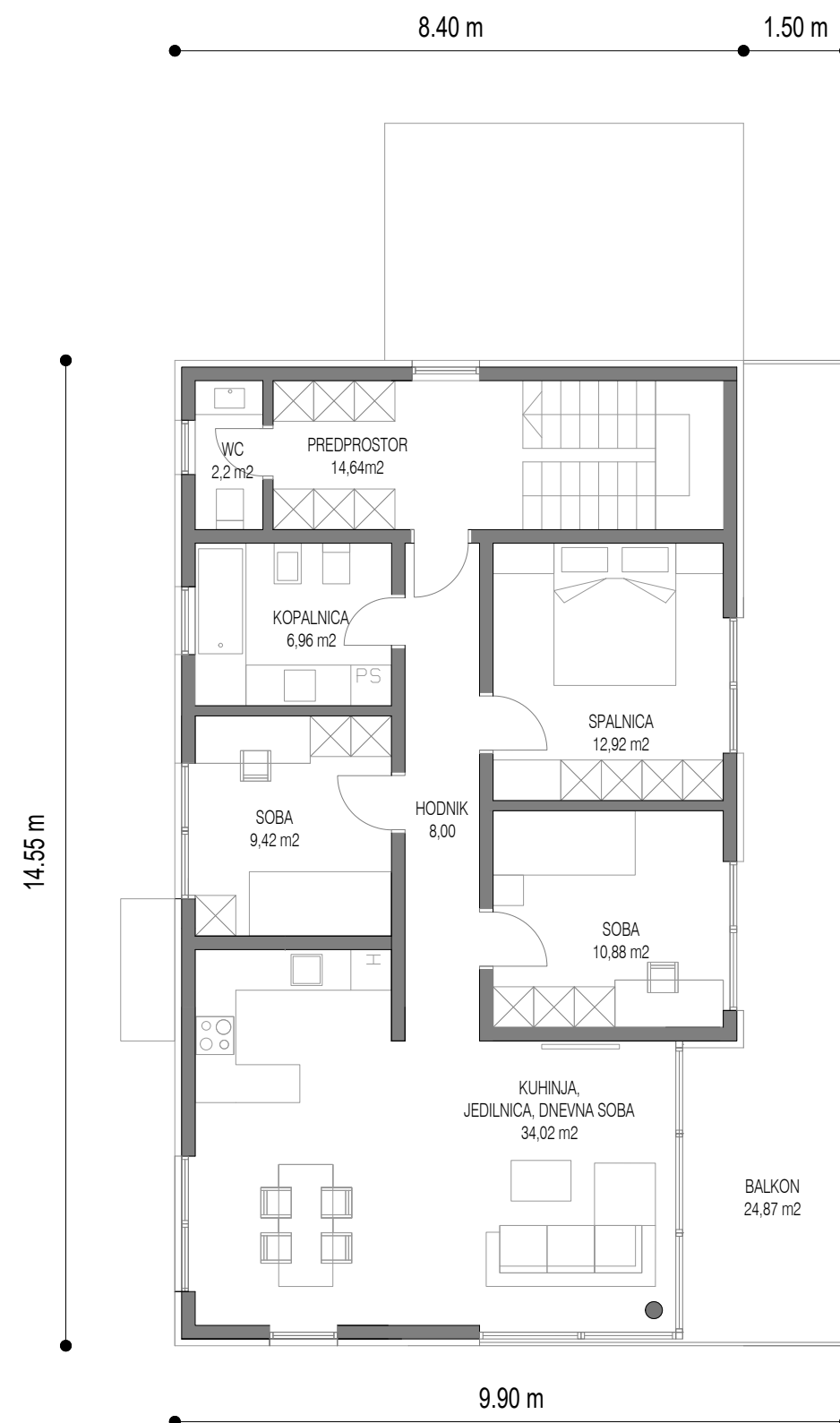
TLORIS NADSTROPJA
