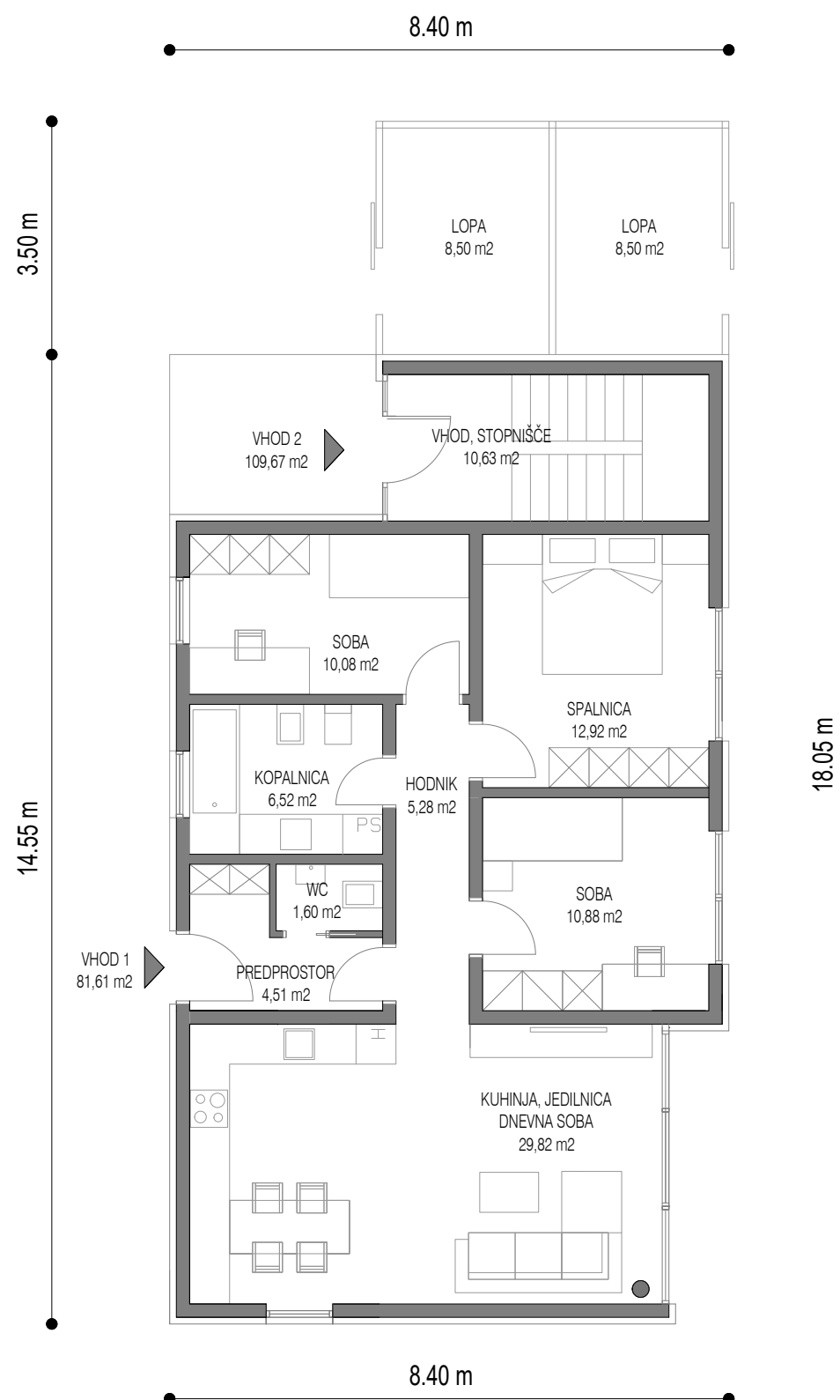
TLORIS PRITLIČJA
