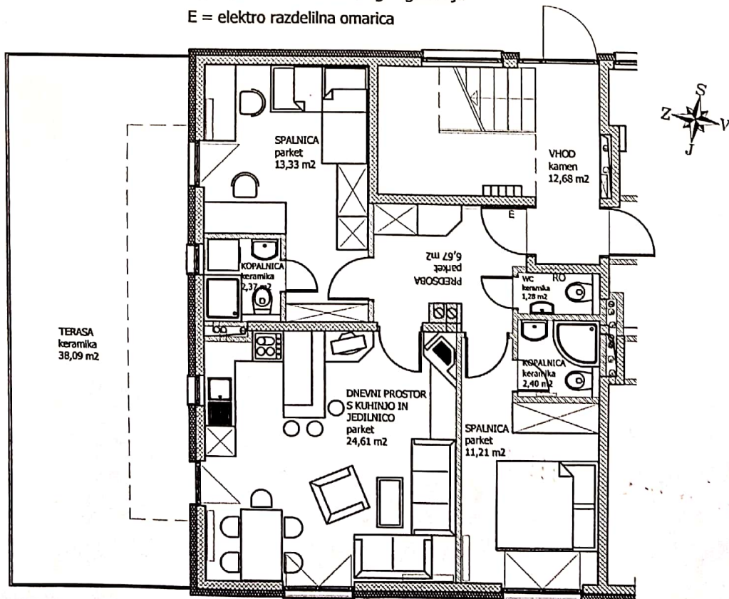
PRITLIČJE objekt A M 1:100
