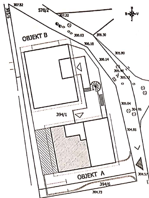
SITUACIJA M 1:500
