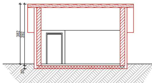
PREREZ D-D M 1:100
