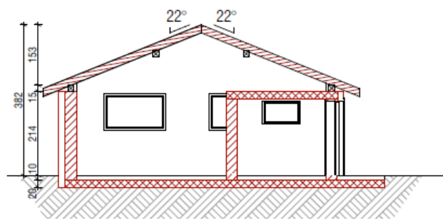
PREREZ C-C M 1:100
